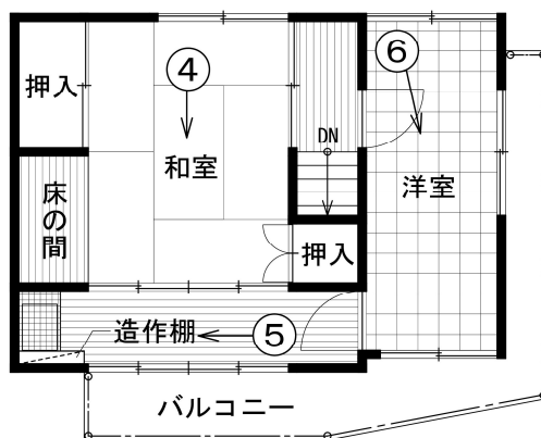
2 階平面図
