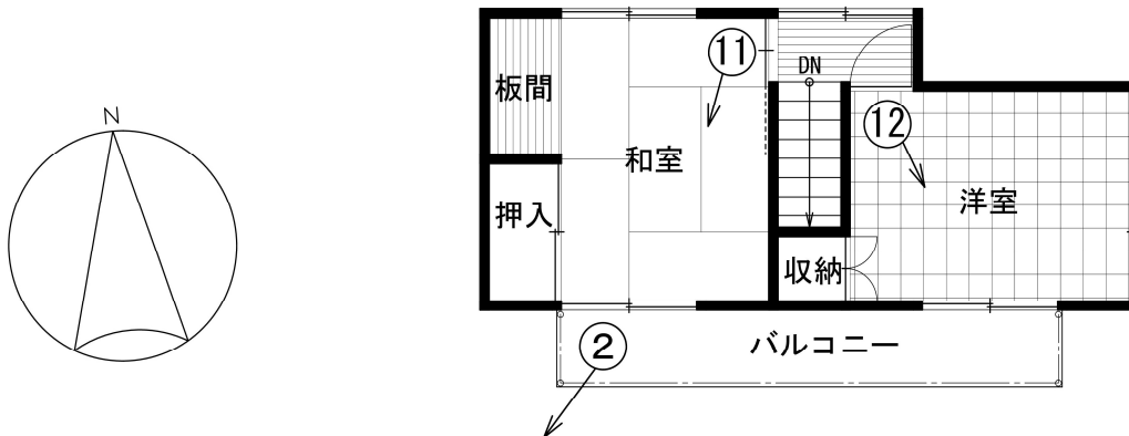
2 階平面図
