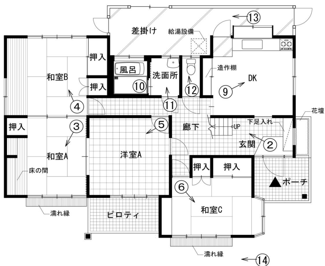
1 階平面図
