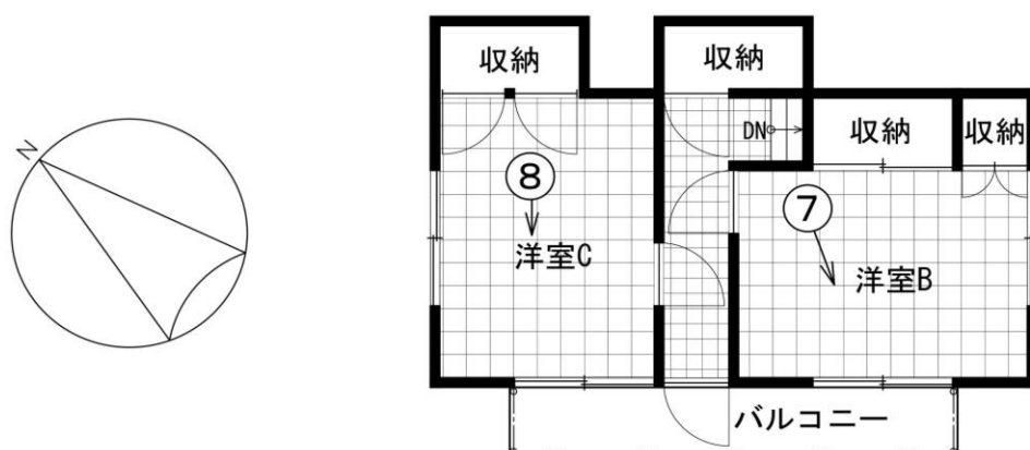
2 階平面図
