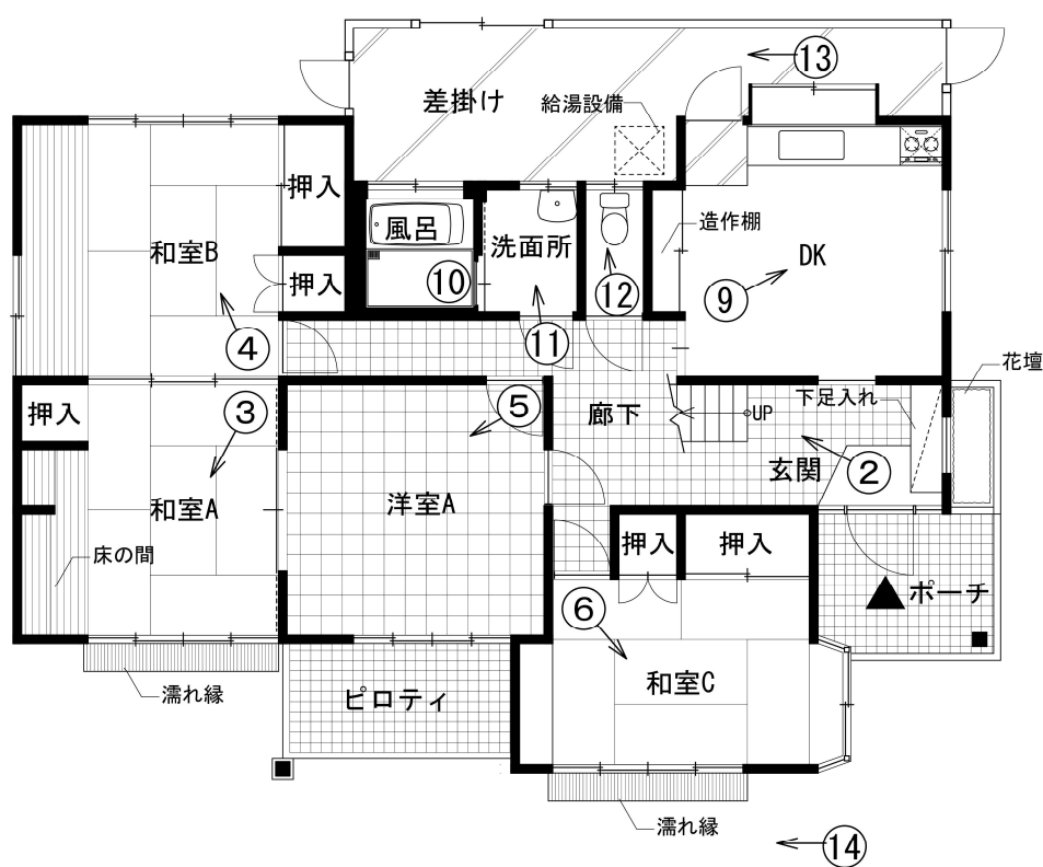
1階平面図
