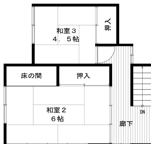
2階平面図
