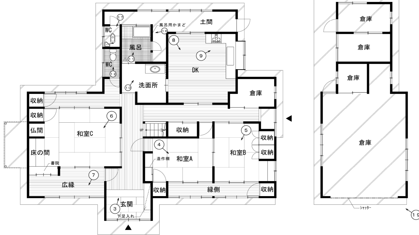
1階平面図
