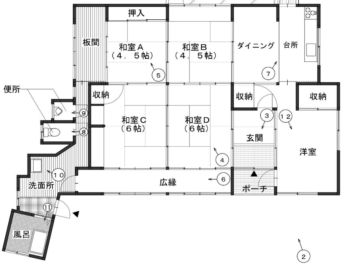
1階平面図
