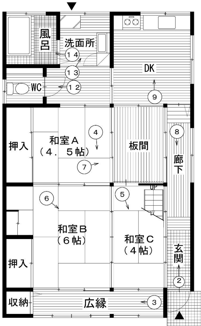
1 階平面図
