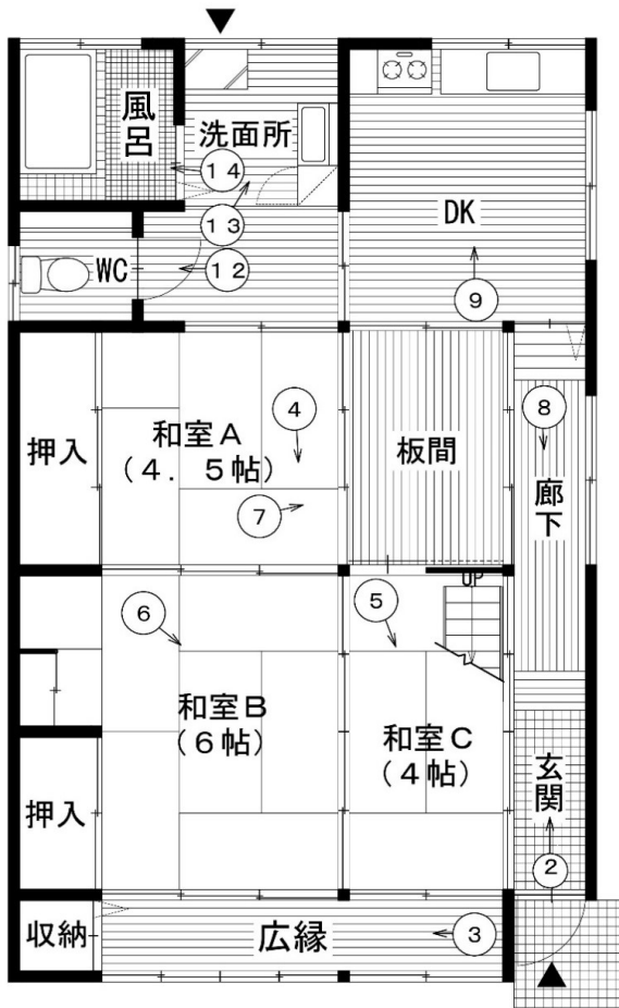
1階平面図
