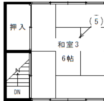
2階平面図
