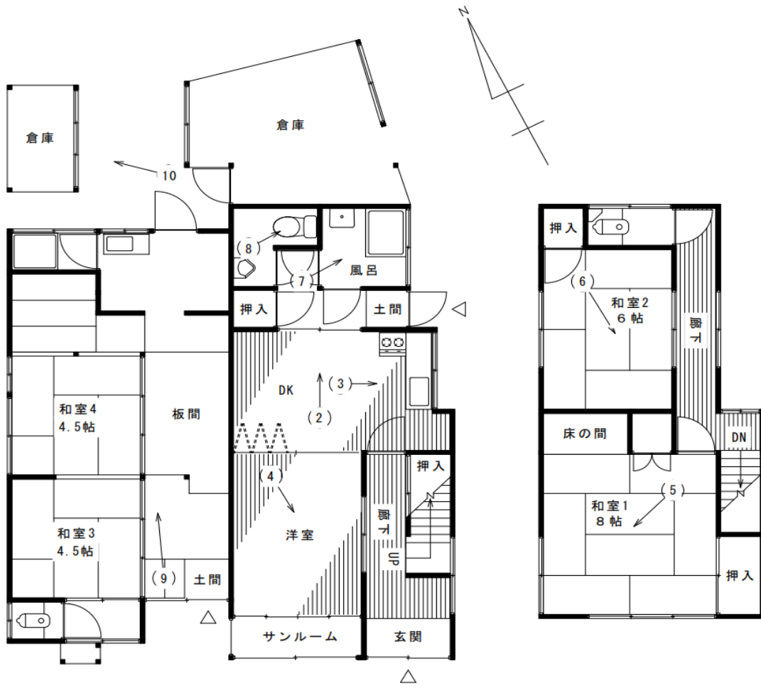
1階平面図
