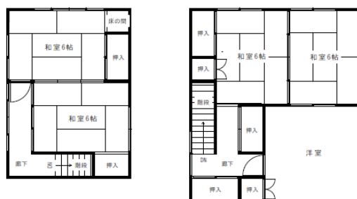
2階平面図
