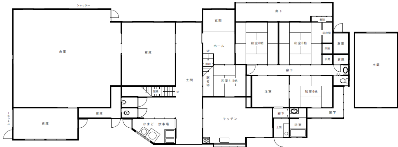
1階平面図
