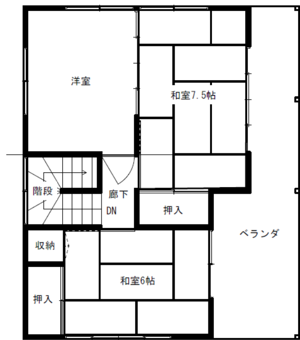
2階平面図
