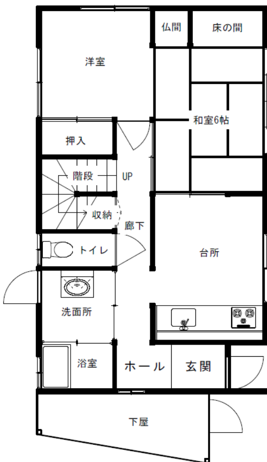
1階平面図
