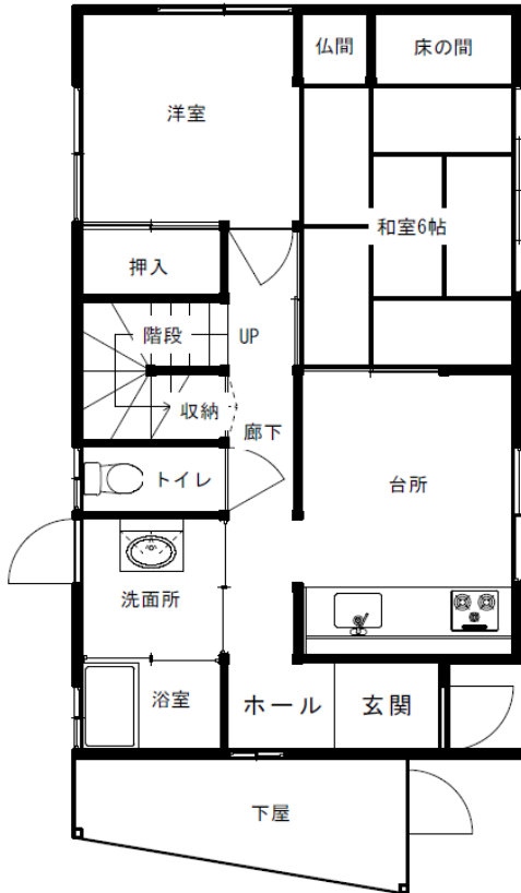
1階平面図
