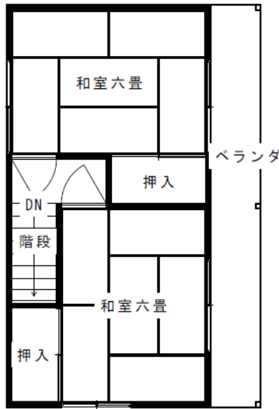
2階平面図
