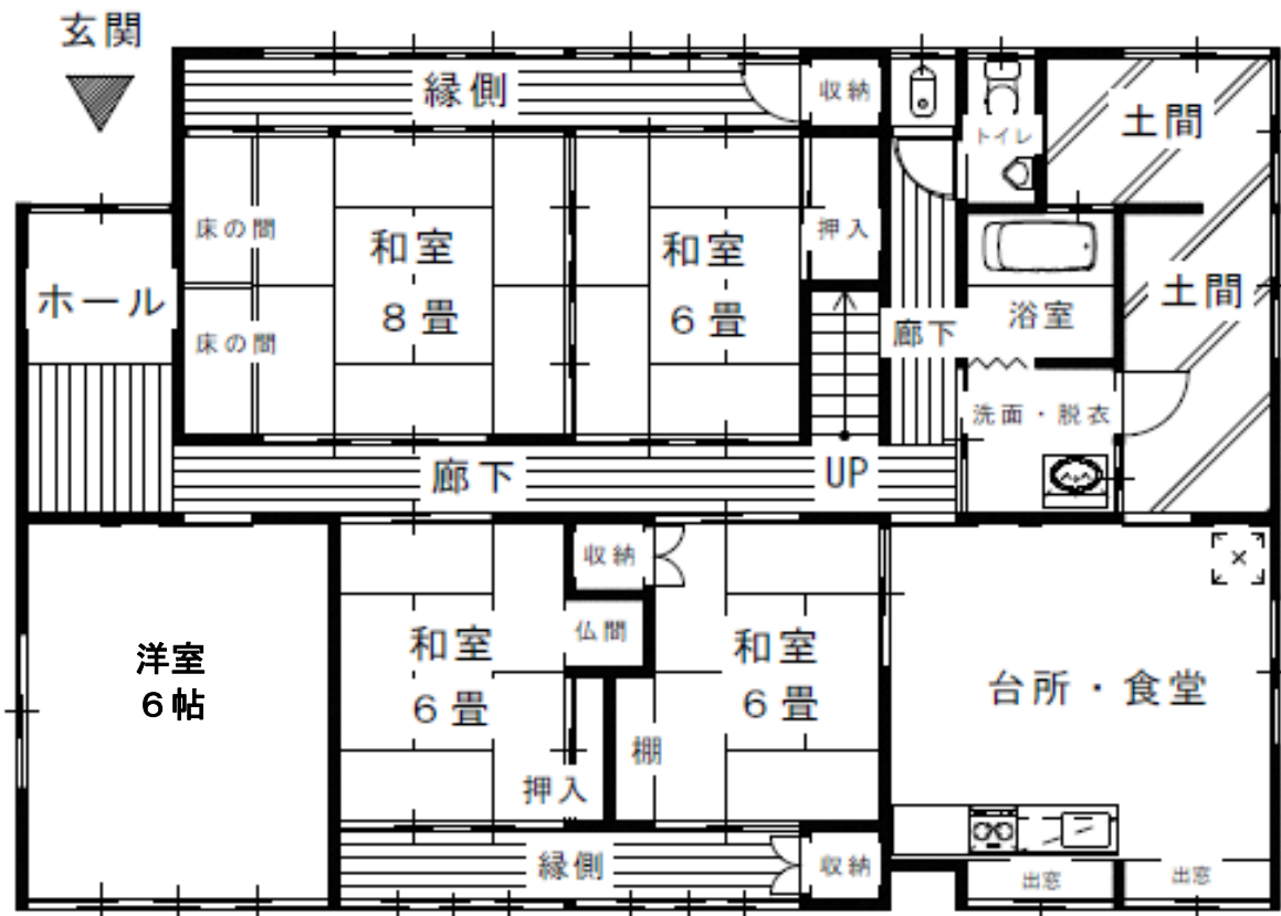
平面図
