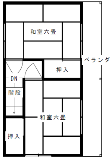
2階平面図
