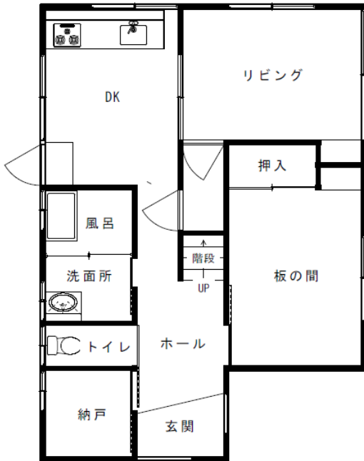
1階平面図
