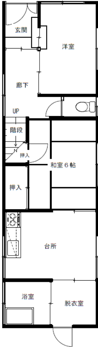
1階平面図
