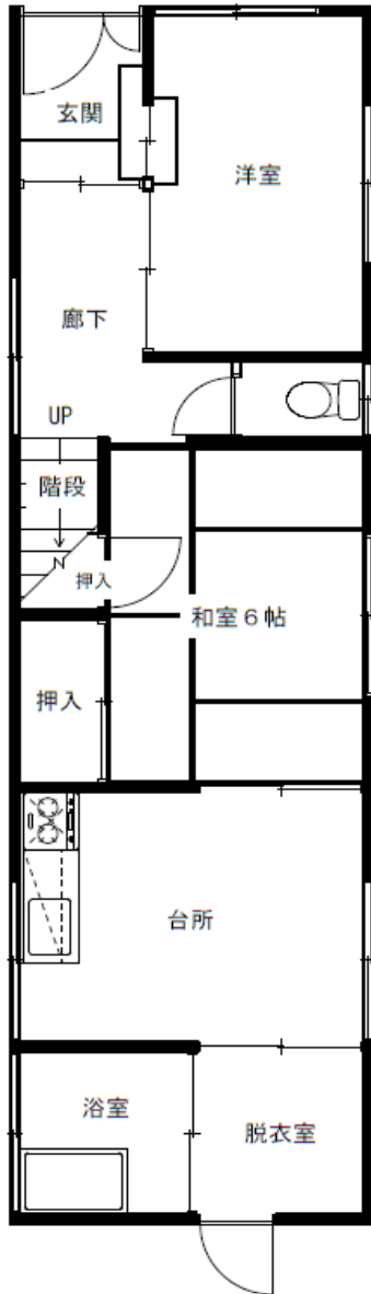
1階平面図
