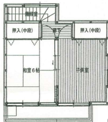
2階平面図
