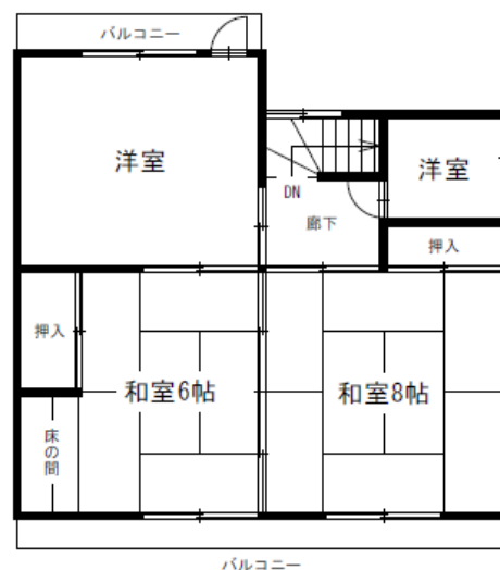
2 階平面図 S=1/100
