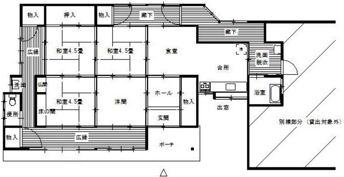
平面図 S=1/100
