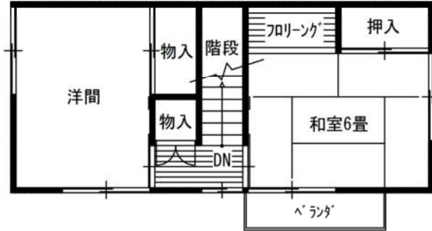
2階平面図 S=1/100
