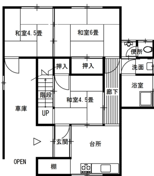
1階平面図 S=1/100
