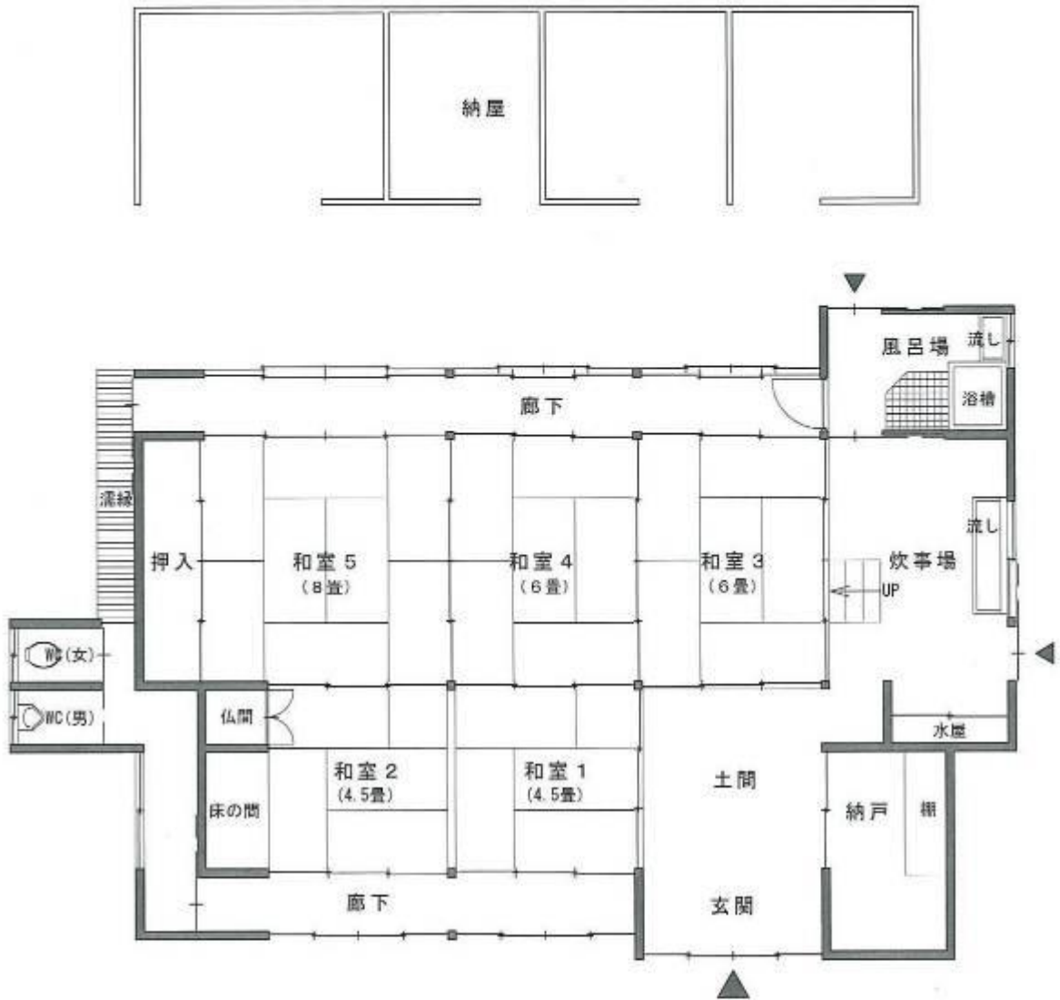
木造住宅平面図 1:100
