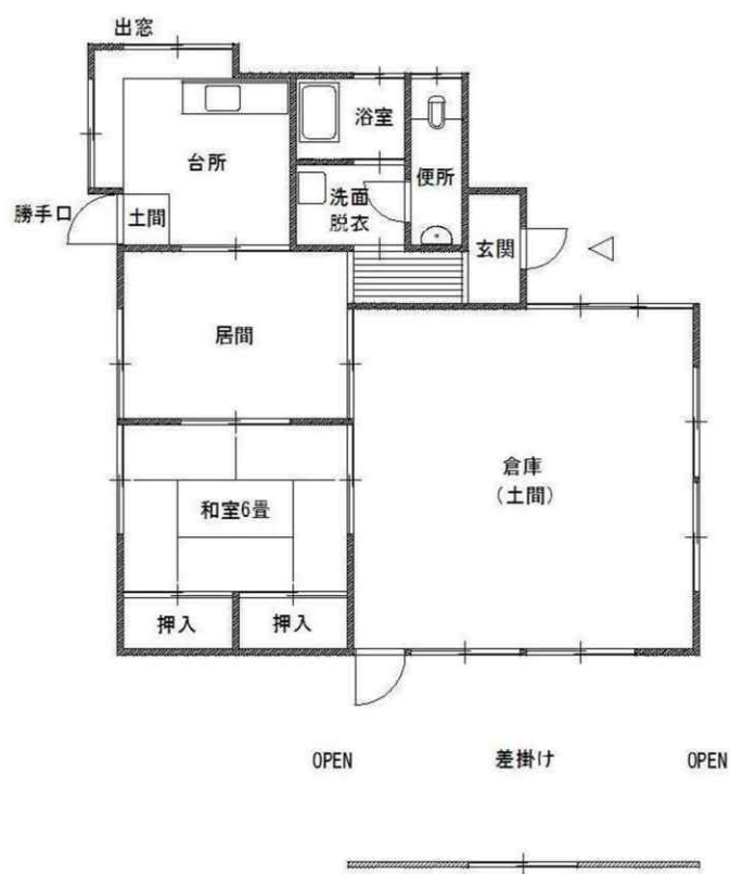
1階平面図 S=1/100
