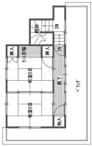
2階平面図 S=1/100
