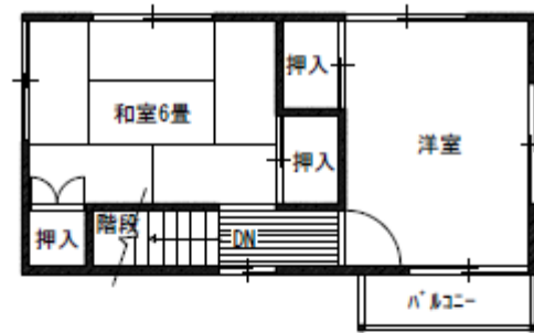
2階平面図 S=1/100
