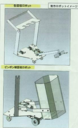
上 缶回収ロボット
